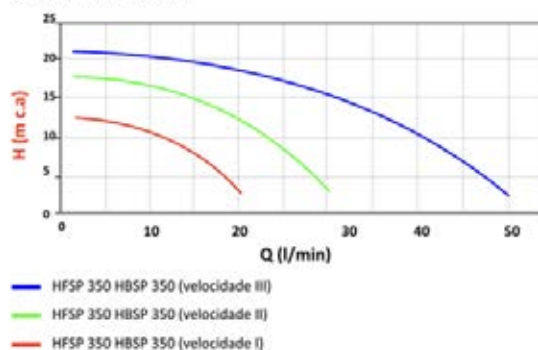
Modelo: HBSP - HFSP 350 Capacidade Máxima = 50 L/min
